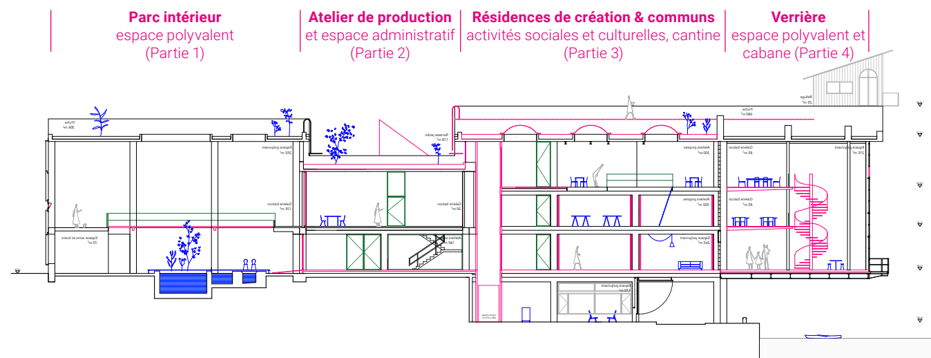
Fig. 14 - Projet de transformation : coupe longitudinale du bâtiment
