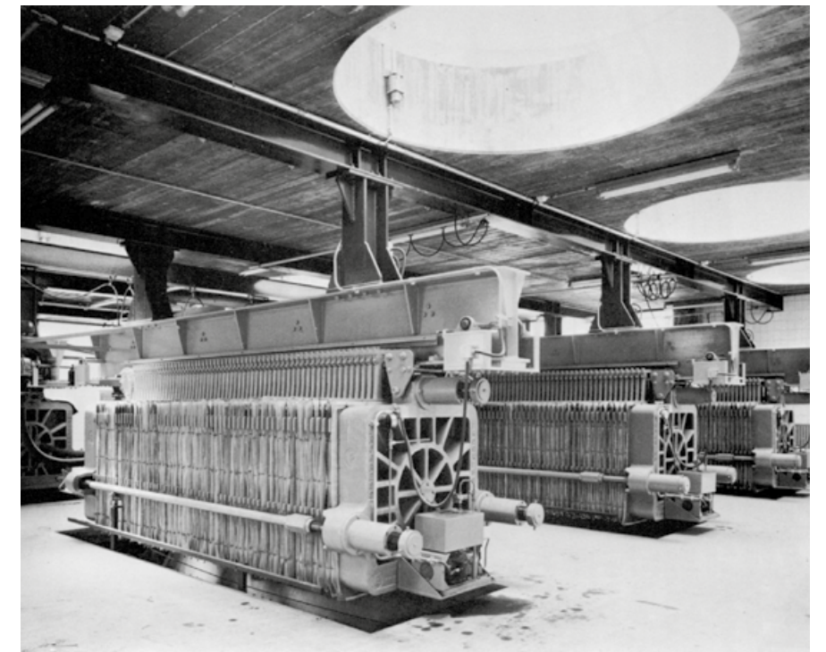
Fig. 12 - Vue des filtre-presses au 2e étage du bâtiment (1967)
