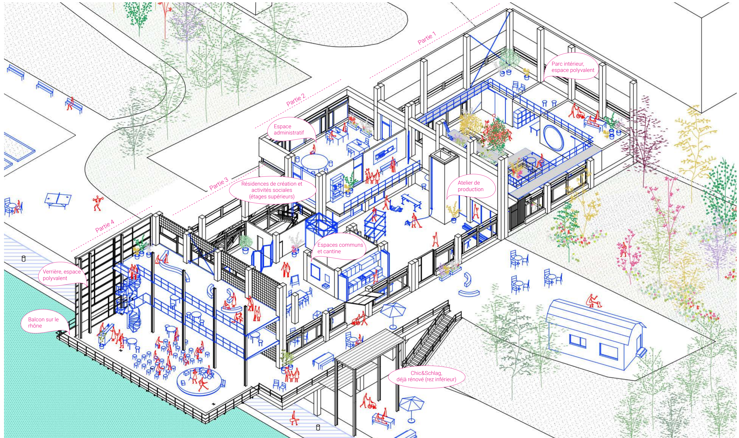
Fig. 33 - Axonométrie du bâtiment avec indications des espaces intérieurs
